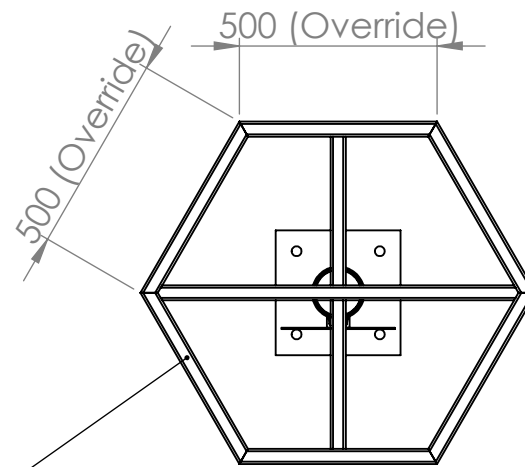
SECTION W-W SCALE 1 : 20
