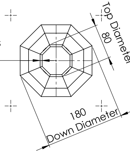
SECTION G-G SCALE 1 : 5
